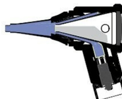
e-scope otoskop światłowodowy
